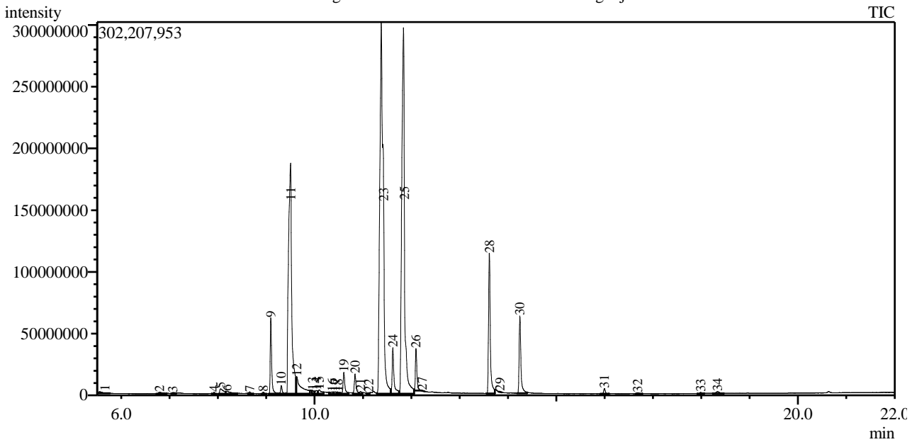
Chromatogram Damasakiniu roziu hidrolatas Bulgarija
